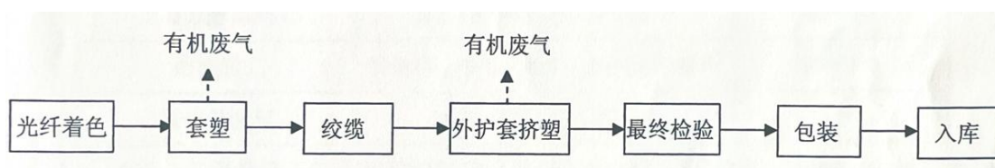
图3-3 生产工艺流程图
